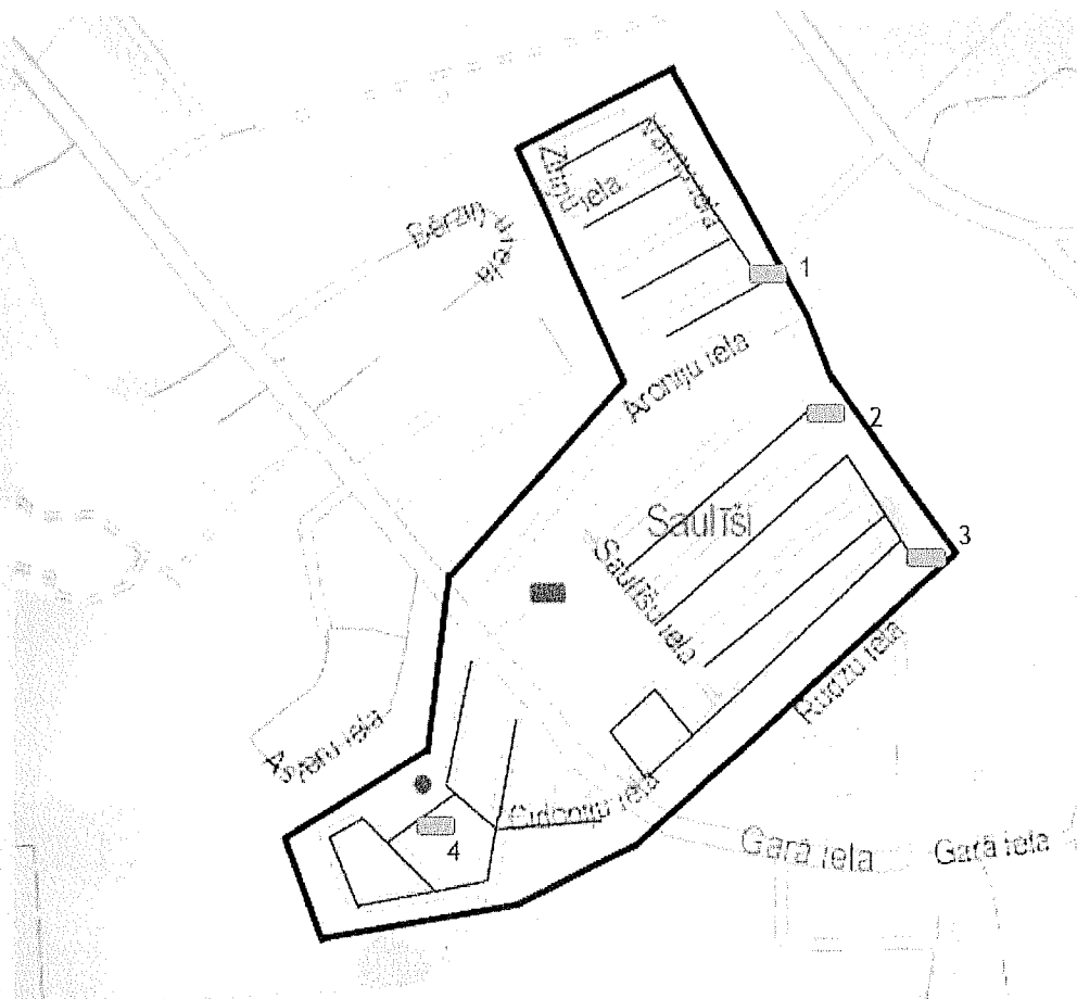
10 attāls: Saulīšu ciemata dzeramā ūdens apgādes un notekūdeņu savākšanas infrastruktūras izvietojums
