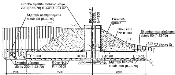
Grēzums 1 - 1
